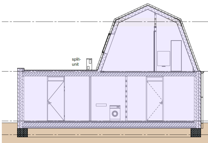
Doorsnede
