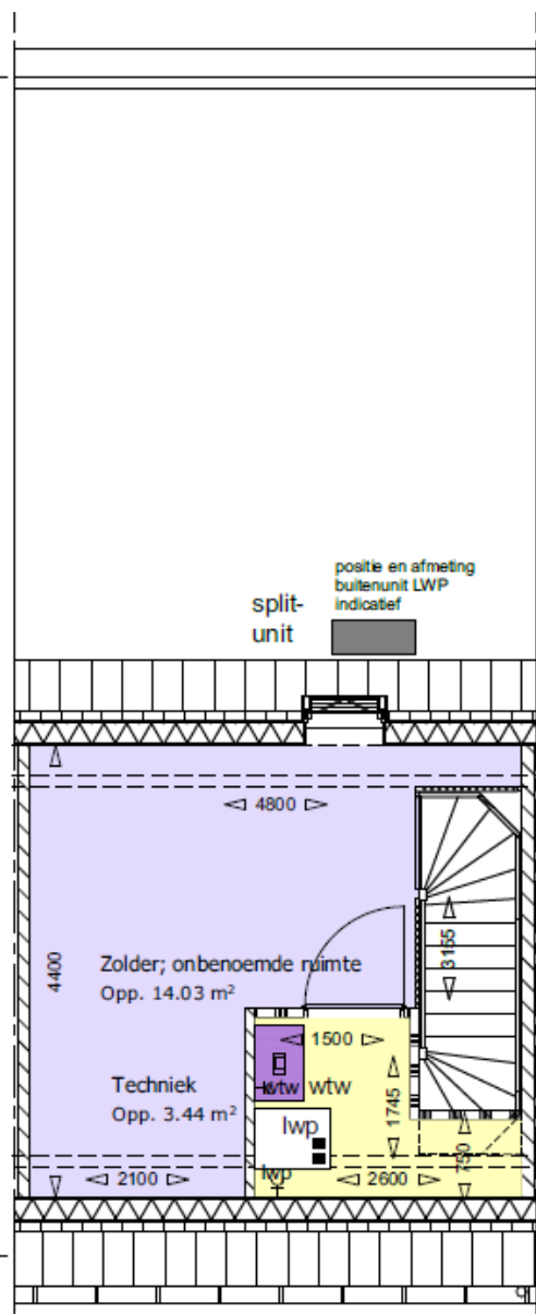
Verdieping
