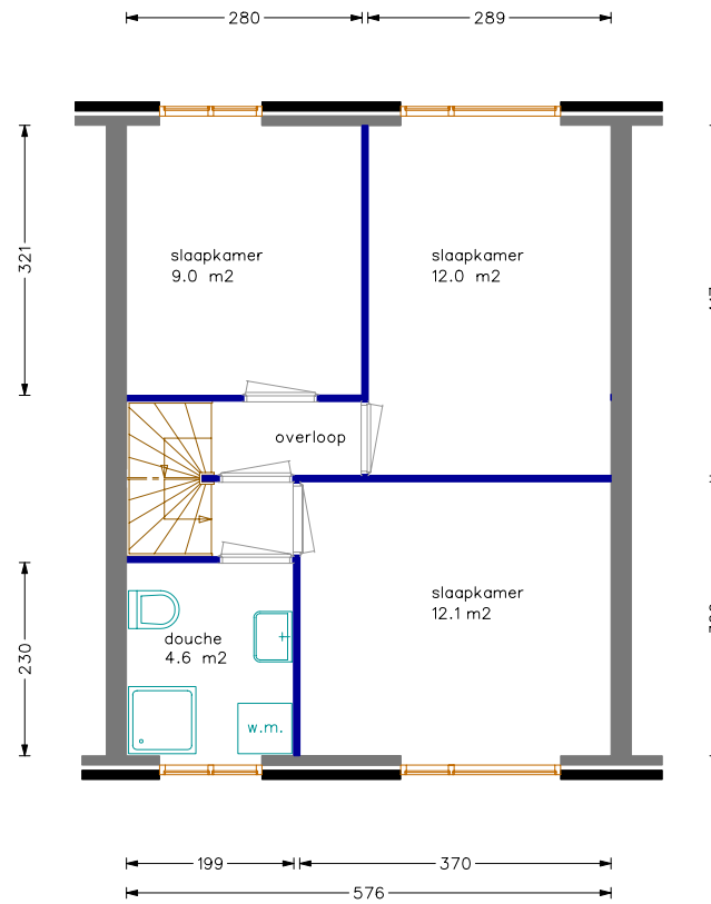
Verdieping
