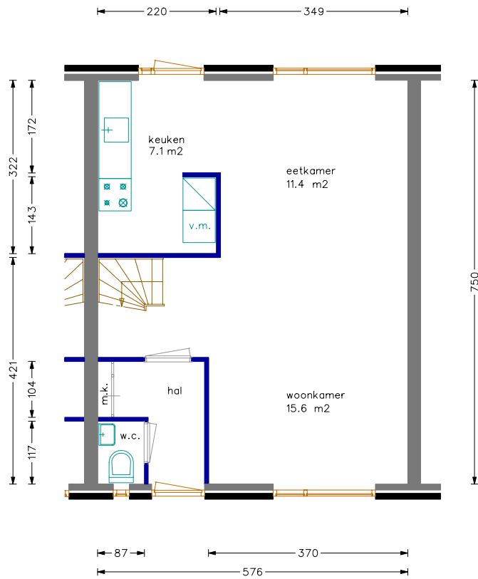
Begane Grond
